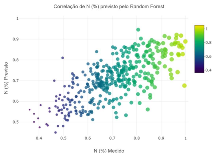
Figura 1. Gráfico de dispersão para os 10 conjuntos (k) de teste pelo método de validação-cruzada.
